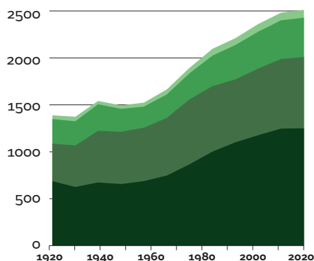
Puuston tilavuus vuosina 1924–2020, miljoonaa m 3 (Suomen nykyrajojen alueella)
